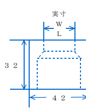
昭和精工用ダイス ※42mm口の四角型
